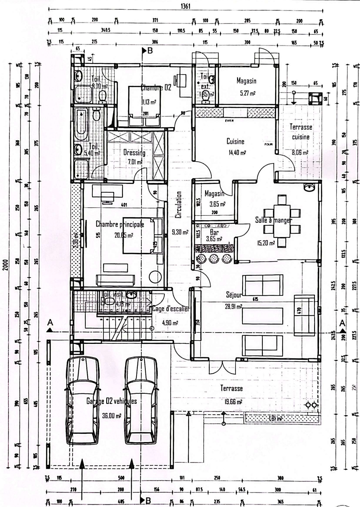
PLAN DE NIVEAU RDC
